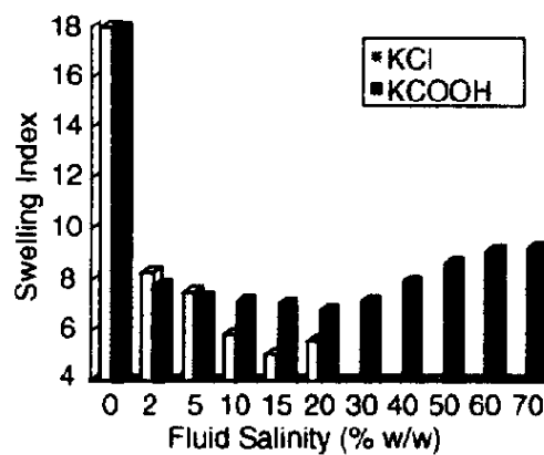
Figure 8-7: Swelling vs. fluid salinity (van Oort, 1997).
