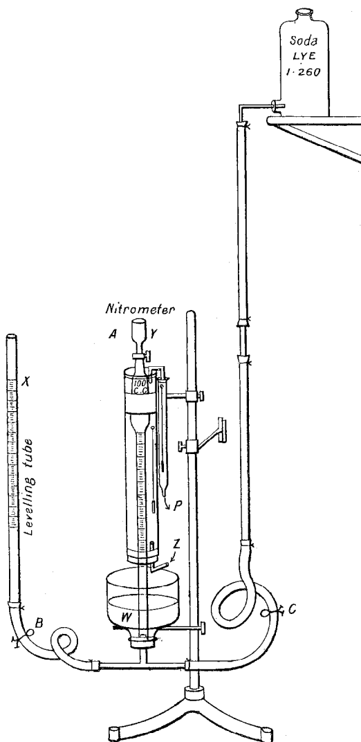
FIG. 44.—SCHULTZE-TIEMAN APPARATUS.
