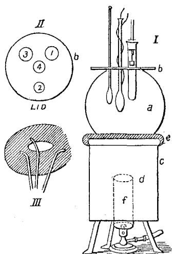
FIG. 46.—HEAT TEST APPARATUS.
