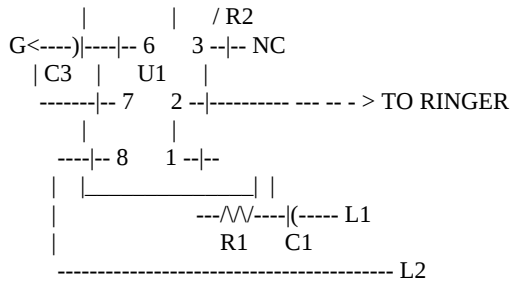
a. Main ringer TTL circuit
