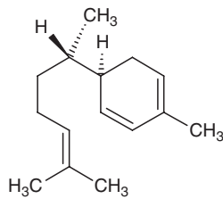
\alpha -Zingiberene
