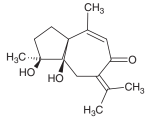
Procumadiol
