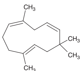
\alpha -Humulene
