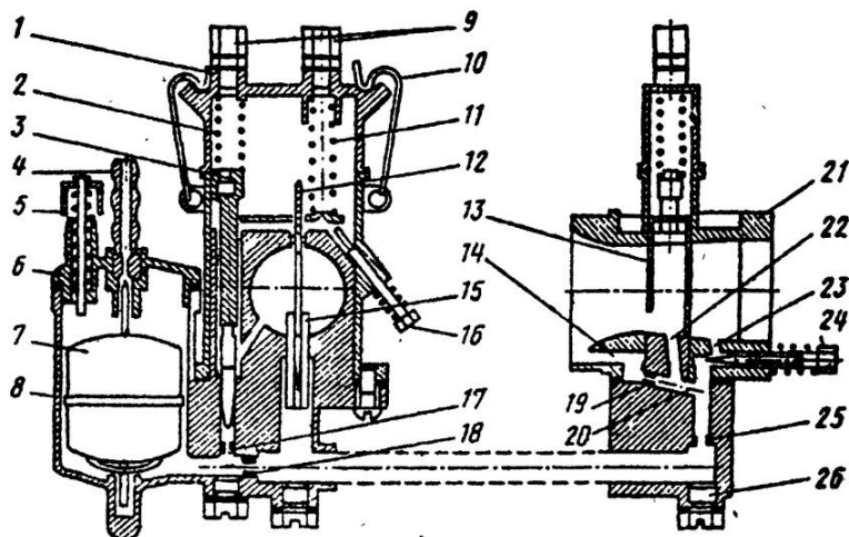
Рис. 3.4. Карбюратор К-36:
