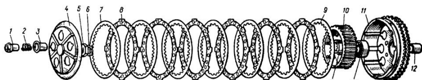
Рис. 5.6. Муфта сцепления мотоциклов "ИЖ-ПЗ", "ИЖ-ПЗ-02", "ИЖ-П4", "ИЖ-П5"
