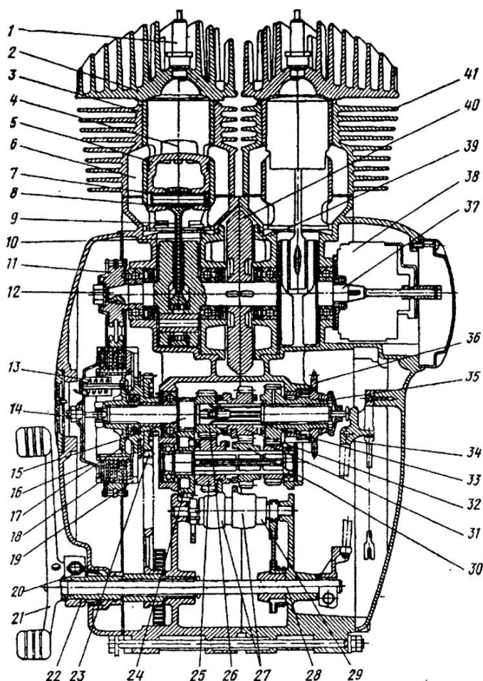
Рис. 2.3. Двигатель "Иж-Ю3" в разрезе:
