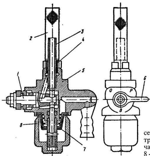
Рис. 3.2. Топливный кран:
