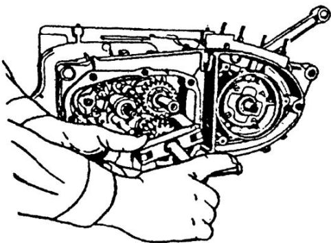
Рис. 5.14. Выпрессовка промежуточного вала "Иж-П5"
