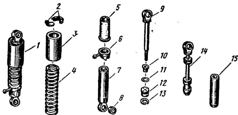
Рис. 6.14. Амортизатор мотоциклов "Иж-Планета-3", "Иж-Планета-3-01", "Иж-Юпитер-3", "Иж-Юпитер-3-01", "Иж-Планета-Спорт" (наименования и количество деталей приведены в табл. 6.8)
