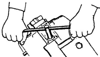
Рис. 5.16. Вывертывание болта крепления выносного маховика “Иж-Ю5”
