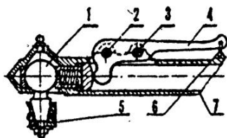
Рис. 6.33. Сцепное устройство
