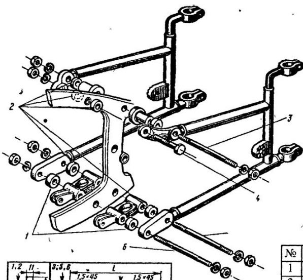
Рис. 6.37. Переделка задней части рамы “Иж-49” и нужные для этого детали:
