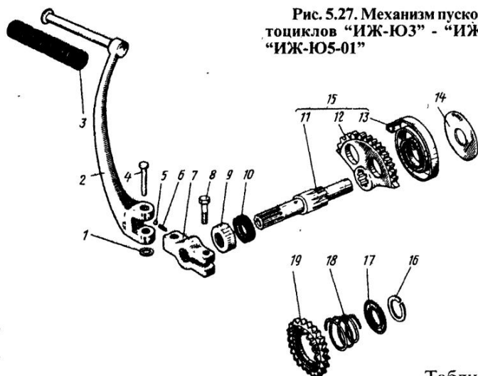
Механизм пусковой мотоциклов "ИЖ-ЮЗ"- "ИЖ-Ю5", "ИЖ-Ю5-01"
