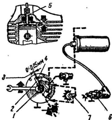
Рис. 7.27. Установка зажигания:
