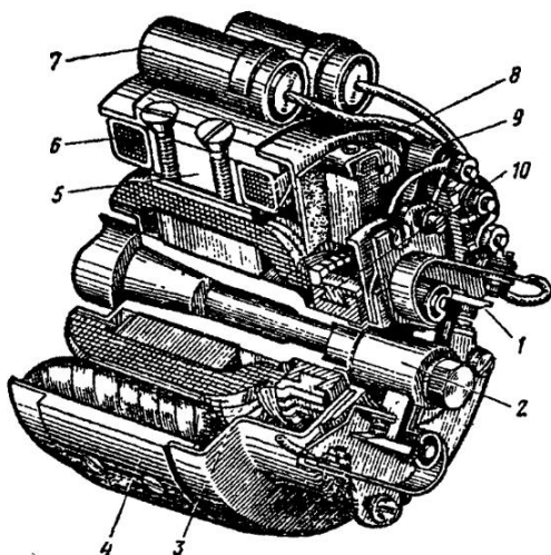
Рис. 7.10. Генератор Г-36М8:
