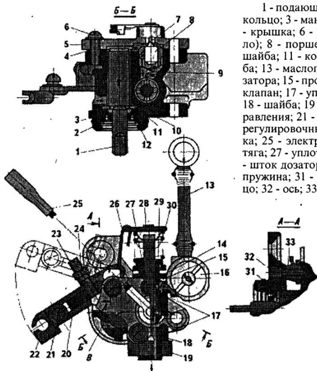
Рис. 3.11. Масляный насос:
