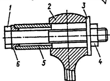
Рис. 2.21. Запрессовка втулки верхней головки шатуна с помощью приспособления:
