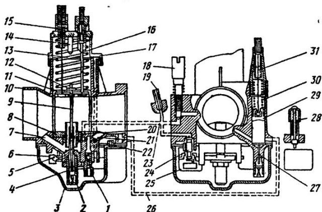
Рис. 3.5. Карбюратор К-62:
