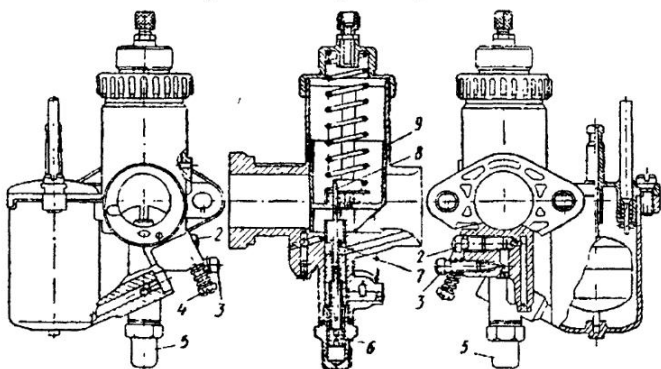
Рис. 3.6. Карбюратор Йиков мотоциклов:
