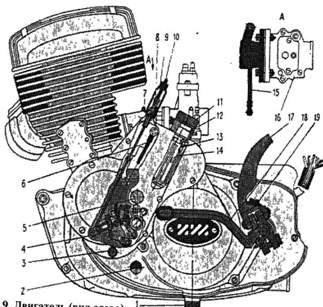
Рис. 3.9. Двигатель (вид слева):
