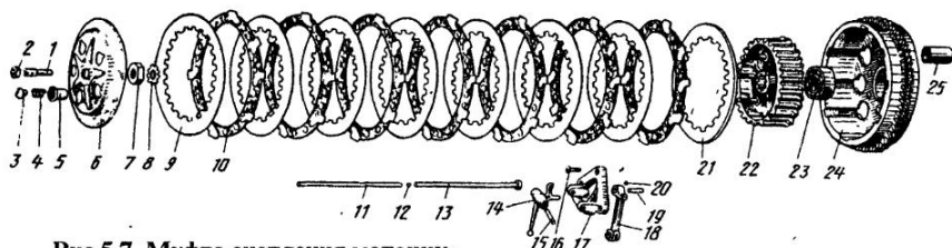
Рис 5.7. Муфта сцепления мотоциклов “ИЖ-Ю3”, “ИЖ-Ю4”, “ИЖ-Ю5”, “ИЖ-Ю5-01”
