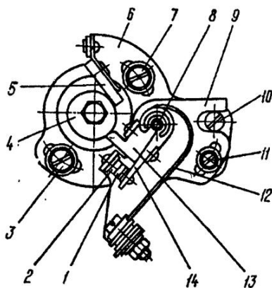
Рис. 7.26. Прерыватель генераторов Г-36М1 и Г-36М7:
