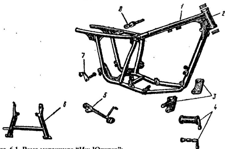
Рис. 6.1. Рама мотоцикла “Иж-Юпитер”:
