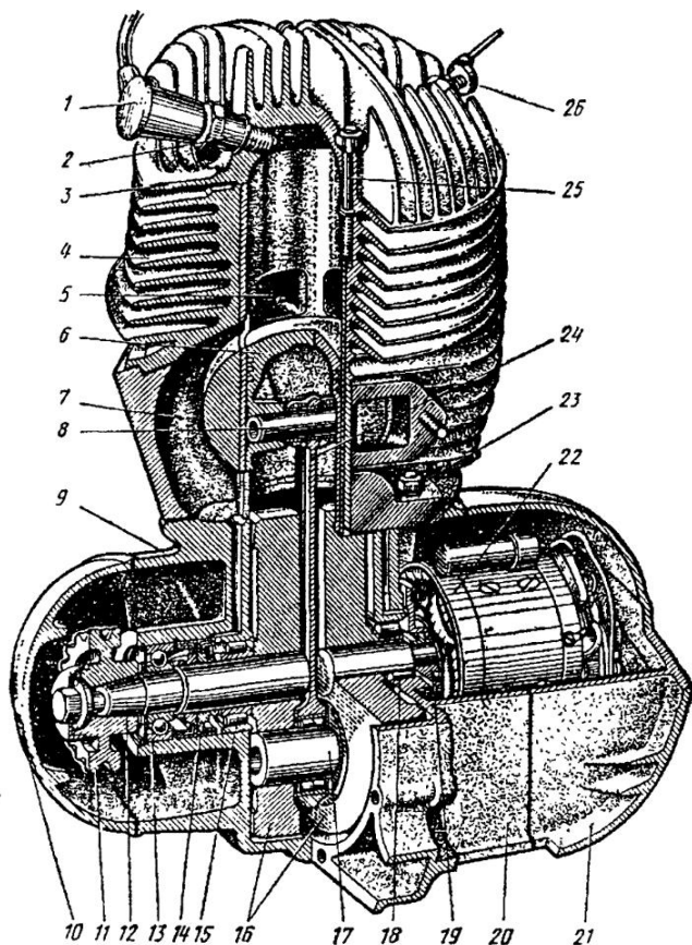
Рис. 2.2. Двигатель "Иж-П2":
