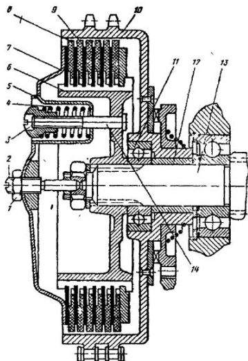
Рис. 5.2. Сцепление мотоцикла "Иж-ЮЗ":
