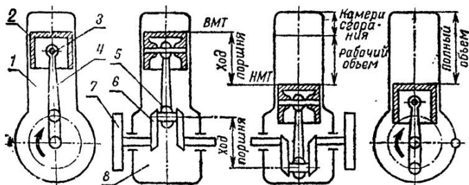
Рис. 2.1. Схема двигателя внутреннего сгорания:
