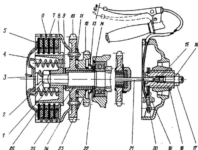
Рис. 5.3. Сцепление:
