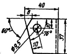
Рис. 7.18. Чертеж кронштейна для установки реле-регулятора ИЖ-PP-1
