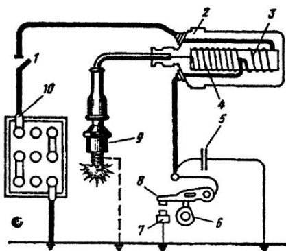
Рис. 7.25. Схема батарейного зажигания:
