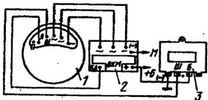
Рис. 7.17. Схема подключения реле-регулятора PP362-Б (или PP362-А) вместо ИЖ-РН-2С:
