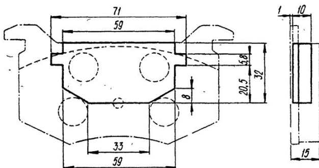
Рис. 6.27. Изготовление тормозной колодки
