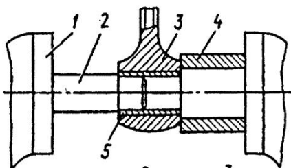
Рис. 2.19. Выпрессовка втулки верхней головки шатуна с помощью тисков: 1 - тиски; 2 - оправка; 3 - шатун; 4 - втулка; 5 - втулка верхней головки шатуна
