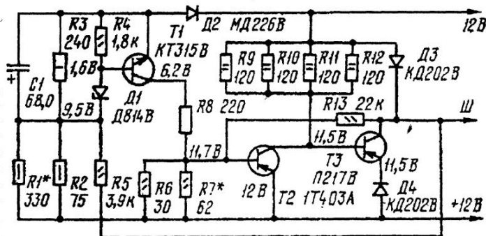
Рис. 7.16. Схема регулятора напряжения Иж-РН-2С: резисторы R1 - R3, R8 - R12 типа МЛТ; резисторы R4 - R7, R13 типа ВС; R1, R7 подбираются при регулировке
