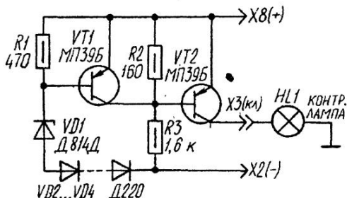
Рис. 7.23. Схема включения контрольной лампы
