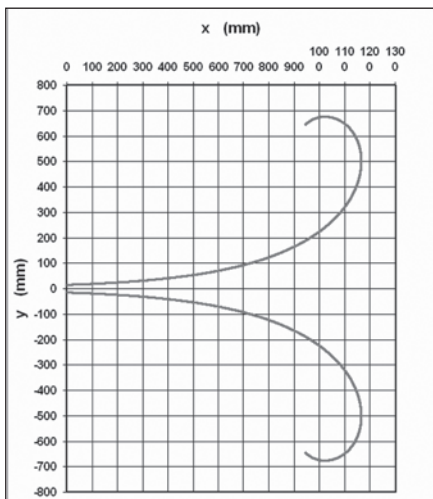
FIGURE 25: Contour of a Le Cléac'h horn.
