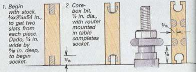
Fig. 5: Shaping the interlocking slats
